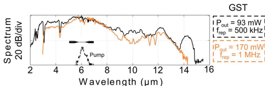
Figure 1 : Spectres SC mesurés en sortie de taper long de 5 cm en verre de chalcogénure (GST) pompé à 6.3 \mu\text{m} [1].
